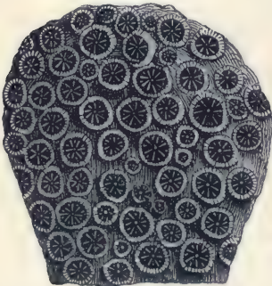
Fig. 379. Astrea tubulosa .
