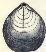
Fig. 242. Radial- streifen.
