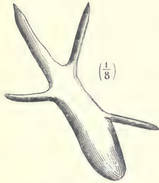
Fig. 50. Tridentipes ingens .
