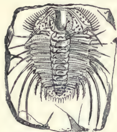
Fig. 144. Odontopl. mira.
