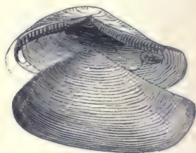
Fig. 292. Nucula Deshayesiana.
