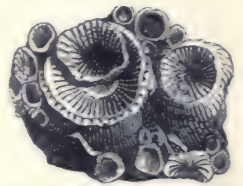
Fig. 383. Cyath. Dianthus.
