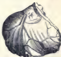
Fig. 221. Terebr. lacunosa .
