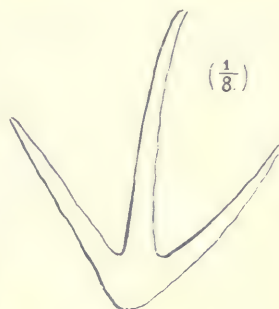
Fig. 49. Argozoum Redfieldi .
