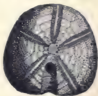
Fig. 322. Nucl. scutatus .
