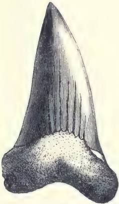
Fig. 84. O. hastalis .
