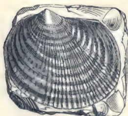
Fig. 281. Posidonia Clarae .
