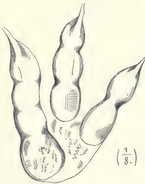
Fig. 47. Brontozoum giganteum .
