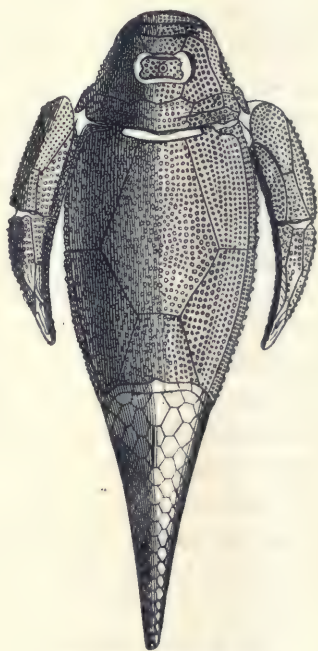
Fig. 116. Pterichthys.
