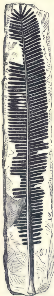
Fig. 428. Pterophyllum Jaegeri .
