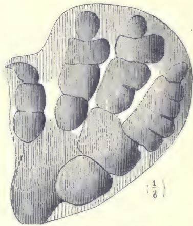
Fig. 48. Otozoum Modii .
