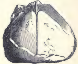
Fig. 225. Pent. Rhenanus .
