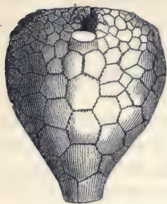
Fig. 362. Mel. hieroglyphicus .
