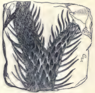
Fig. 421. Lepidodendron Sternbergii .
