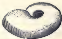
Fig. 176. A. carachtheis .
