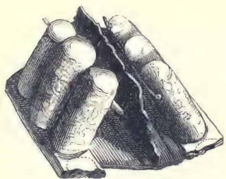
Fig. 57. Phytosaurus cylindricodon .
