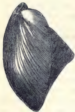
Fig. 285. Cong. subglobosa.
