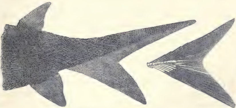
Fig. 94. Homocerci.
